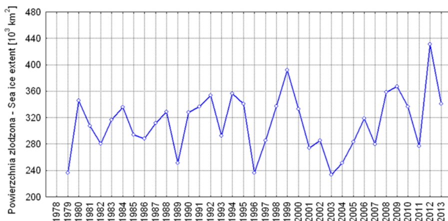
Ryc. 17. Przebieg rocznych wartości powierzchni złodzonej na Morzu Beringa (1979-2013)
