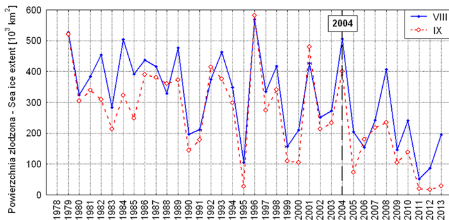
Ryc. 10. Zmiany powierzchni zlodzonej na Morzu Łaptiewów w miesiącach minimum rozwoju powierzchni zlodzonej (sierpień, wrzesień) w latach 1979-2013
