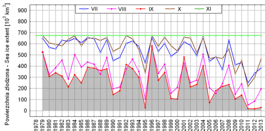
Ryc. 9. Zmiany średniej miesięcznej powierzchni zlodzonej na Morzu Łaptiewów w sezonie nawigacyjnym (lipiec-listopad) w latach 1978-2013
